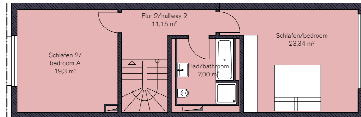
1. Obergeschoss
