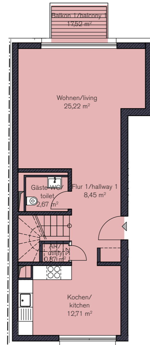
3. Obergeschoss
