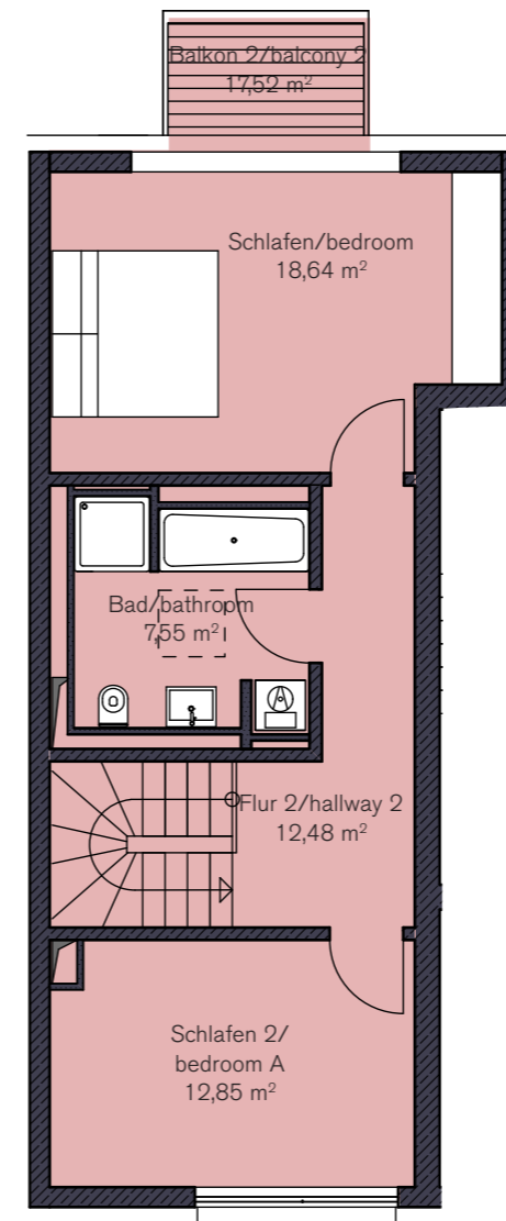
4. Obergeschoss
